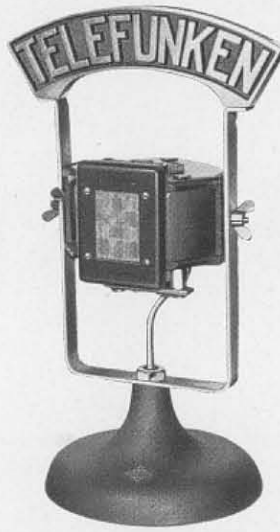
Bild 26, 27, 28. Telefunken-Bändchenmikrofon auf Ständern. Rechts mit Windschutz.
