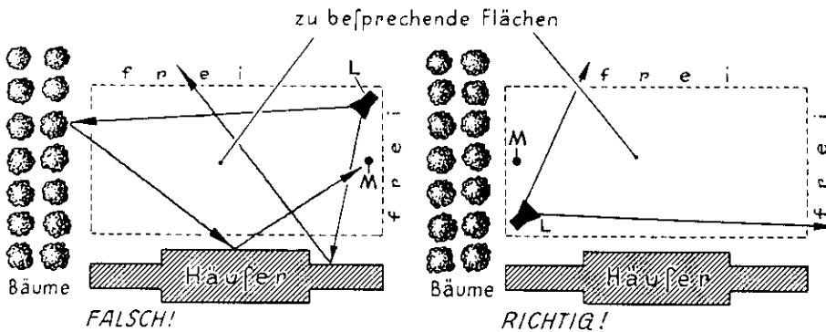
Bild 59. Richtige Aufstellung von Mikrofon und Lautsprechern bei Nähe von echoverursachenden Gegenständen.
