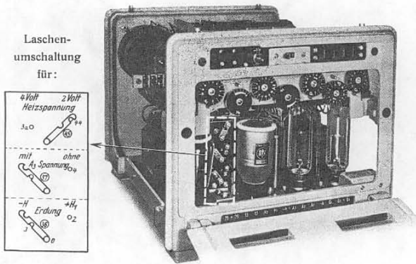
Innenansicht bei abgenommenem Gehäuse
