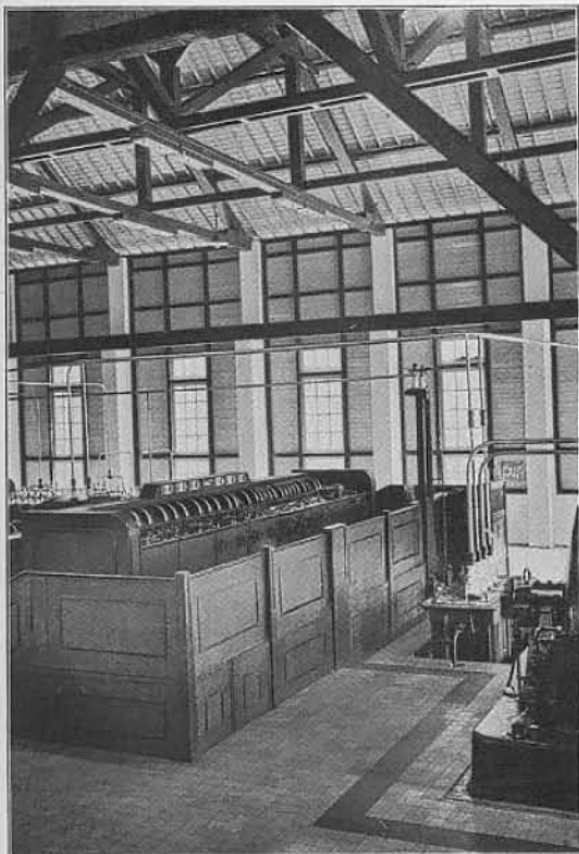
Bild 12. Malabar (Java). Blick auf das Senderbedienungspult für den Maschinensender.
