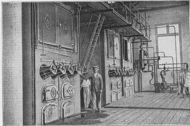
Bild 22. Malabar (Java). Dampfkraftwerk Dajeuhkolot: Die Dampfkesselanlage.
