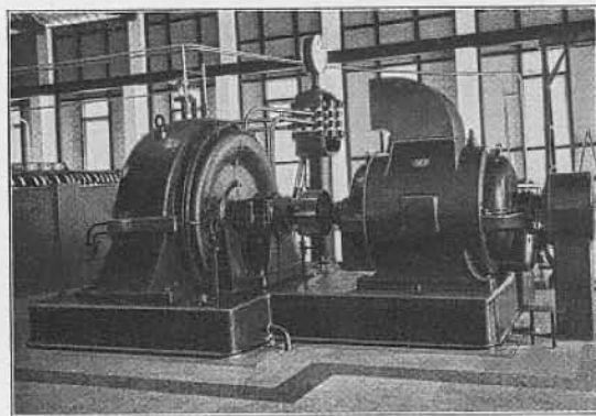
Bild 13. Malabar (Java). 400 MK-Hochfrequenzmaschine mit Antriebsmotor.
