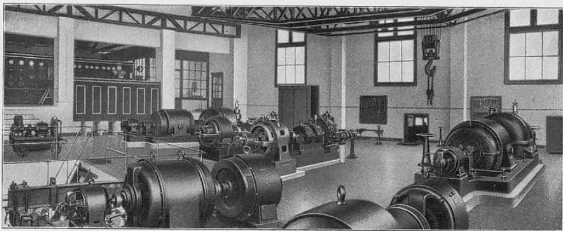
Bild 18. Malabar (Java). Blick in den Turbinensaal des Dampfkraftwerkes Dajuehkolot.
