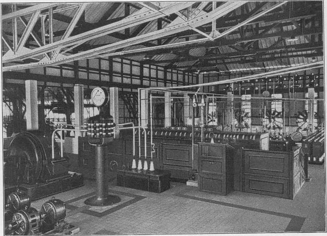
Bild 14. Malabar (Java). Blick in den Maschinensendraum.
