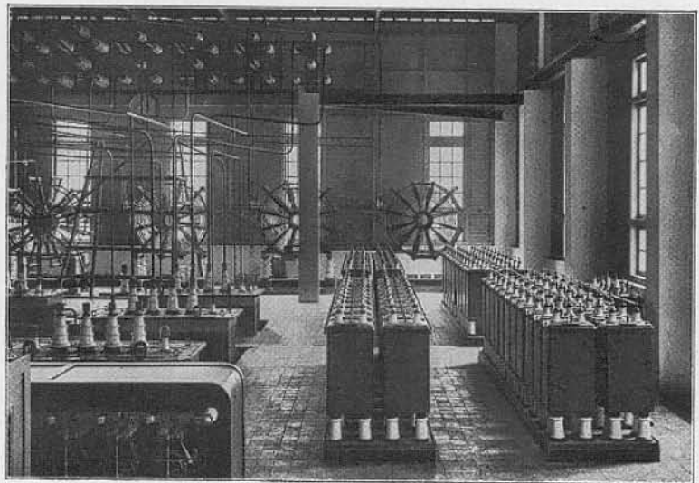
Bild 16. Malabar (Java). Ansicht des Senderraumes.
