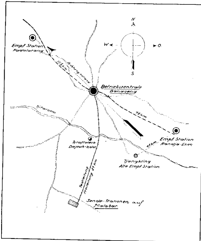
Bild 24. Übersichtskarte über die zu Malabar-Radio gehörigen verschiedenen Betriebsstellen.
