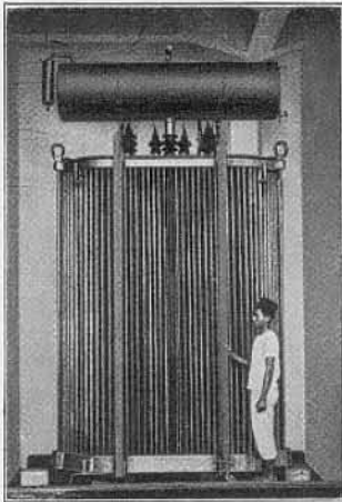
Bild 21. Malabar (Java). Dampfkraftwerk Dajeuhkolot: Transformator in der Unterstation.
