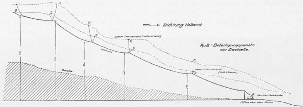
Längsschnitt durch die Malabarschlucht mit Bergantenne.
