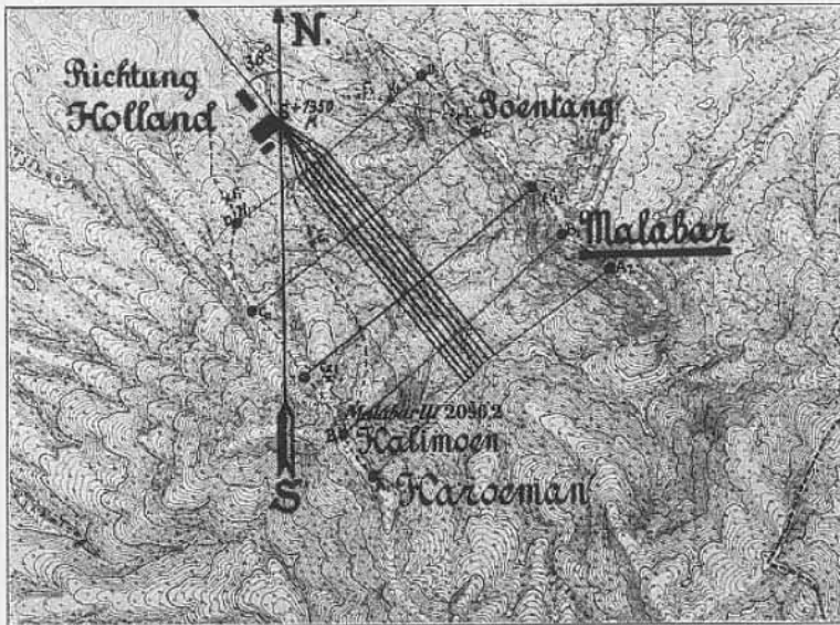
Bild 8. Malabar (Java). Lageplan der Bergantenne in der Schlucht.
