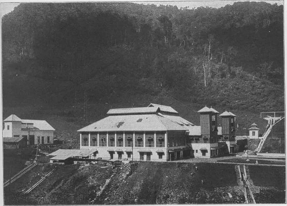
Bild 9. Malabar (Java). Blick auf das Maschinensenderhaus, links die Transformatorenunterstation.
