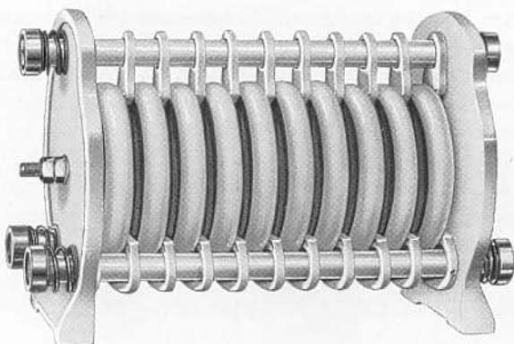
Abbildung 26 Kondensatorblock in Serienschaltung (S-Block)
