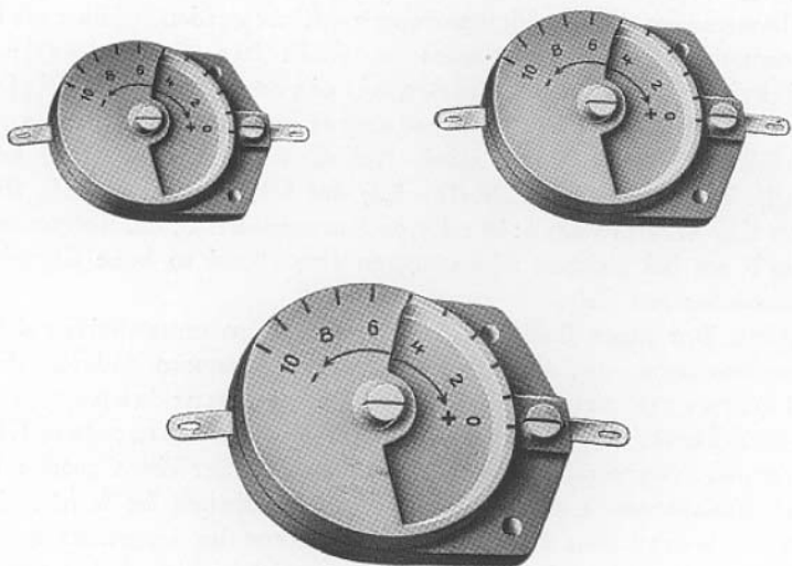
Abbildung 36 Hescho-Temperaturgang-Regler
