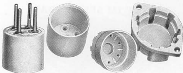
Abbildung 17 Fassungen und Sockel aus Calit für Empfängerröhren
