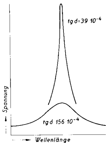
Abbildung 13 Resonanzkurve eines Schwingungskreises mit hohen und eines mit geringen Dämpfungsverlusten
