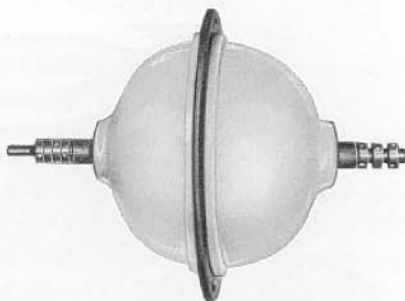
Abbildung 23 HF-Calit-Doppeldurchführung
