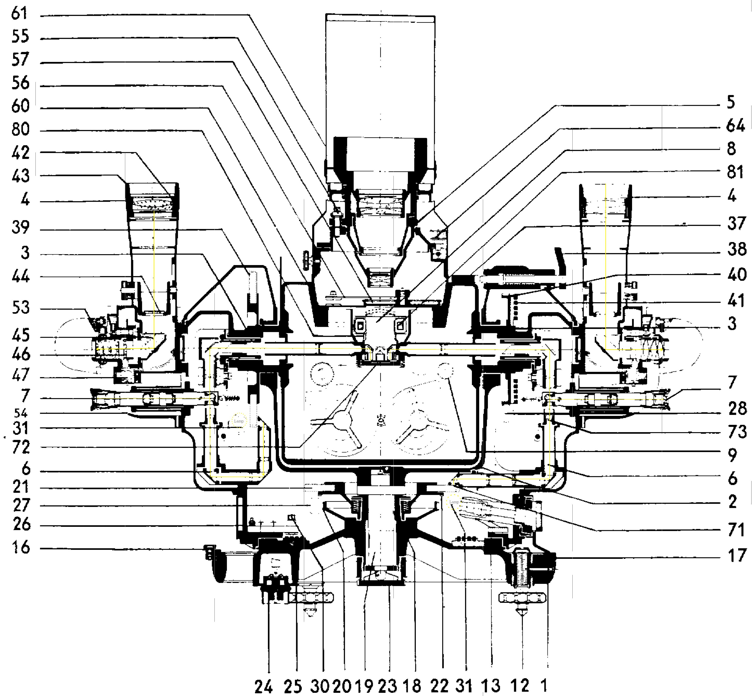
Zeichnung 2. Kinotheodolit-Schnittzeichnung
