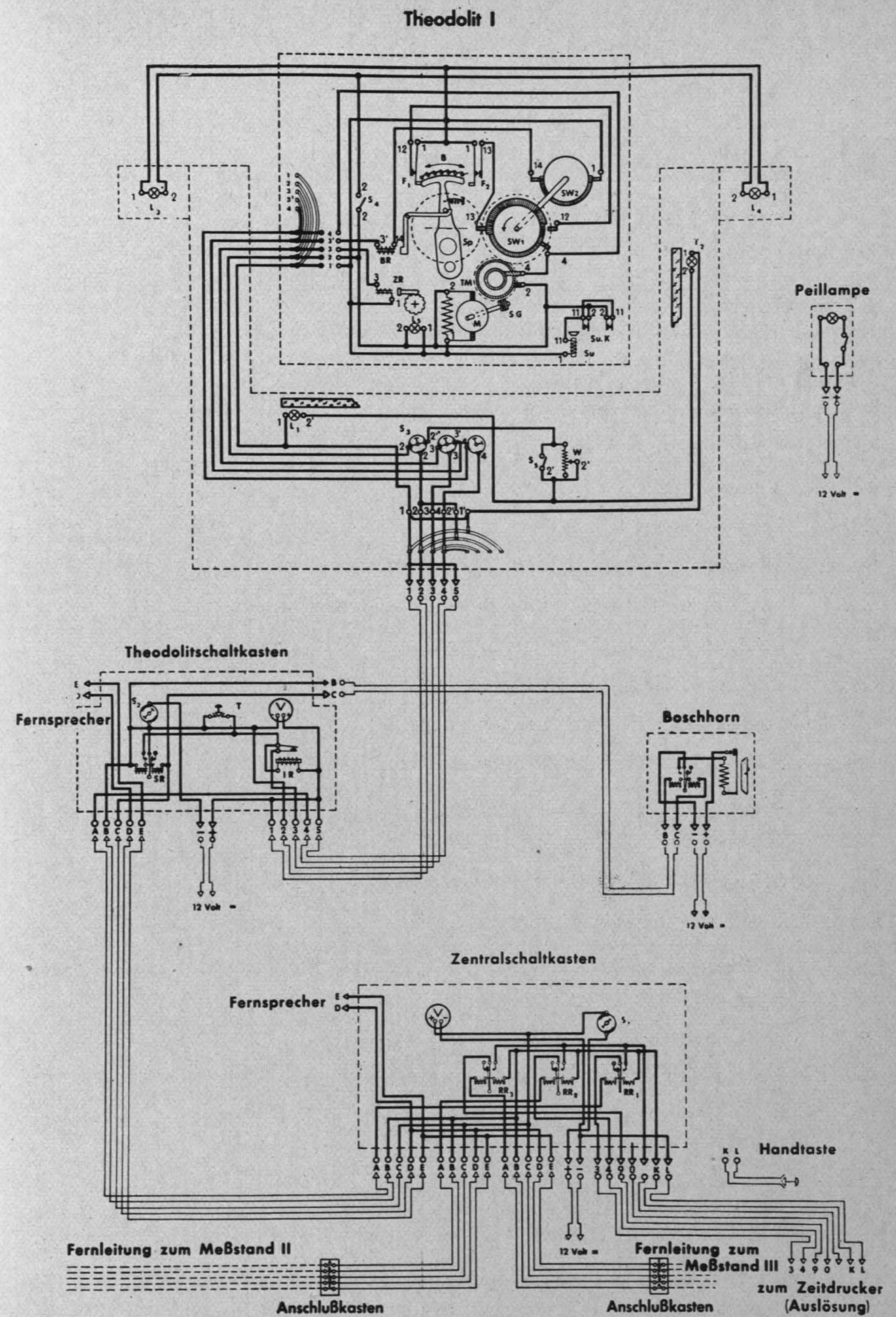
Zeichnung 10. Schaltplan der Kinotheodolit-Meßstation
