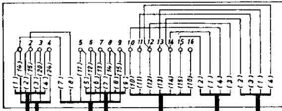
Klemmenkasten III
