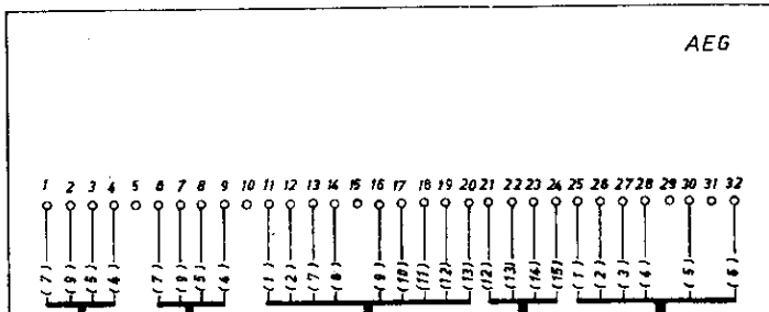
Verstärkerkasten Vk 10a
