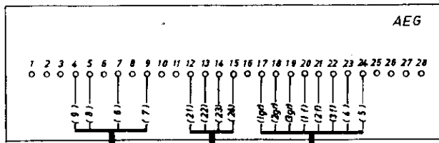
Sollgeber-Höhe
