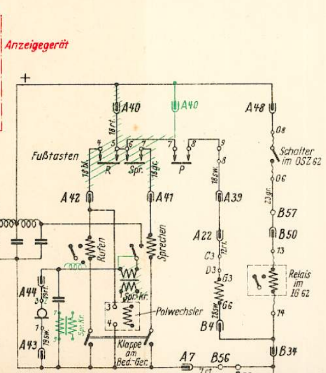
Schaltbild für FuSE 62 A Zusätze für FuSE 62 C, W. Zusätze für FuSE 62 D, D 1, D 2.
