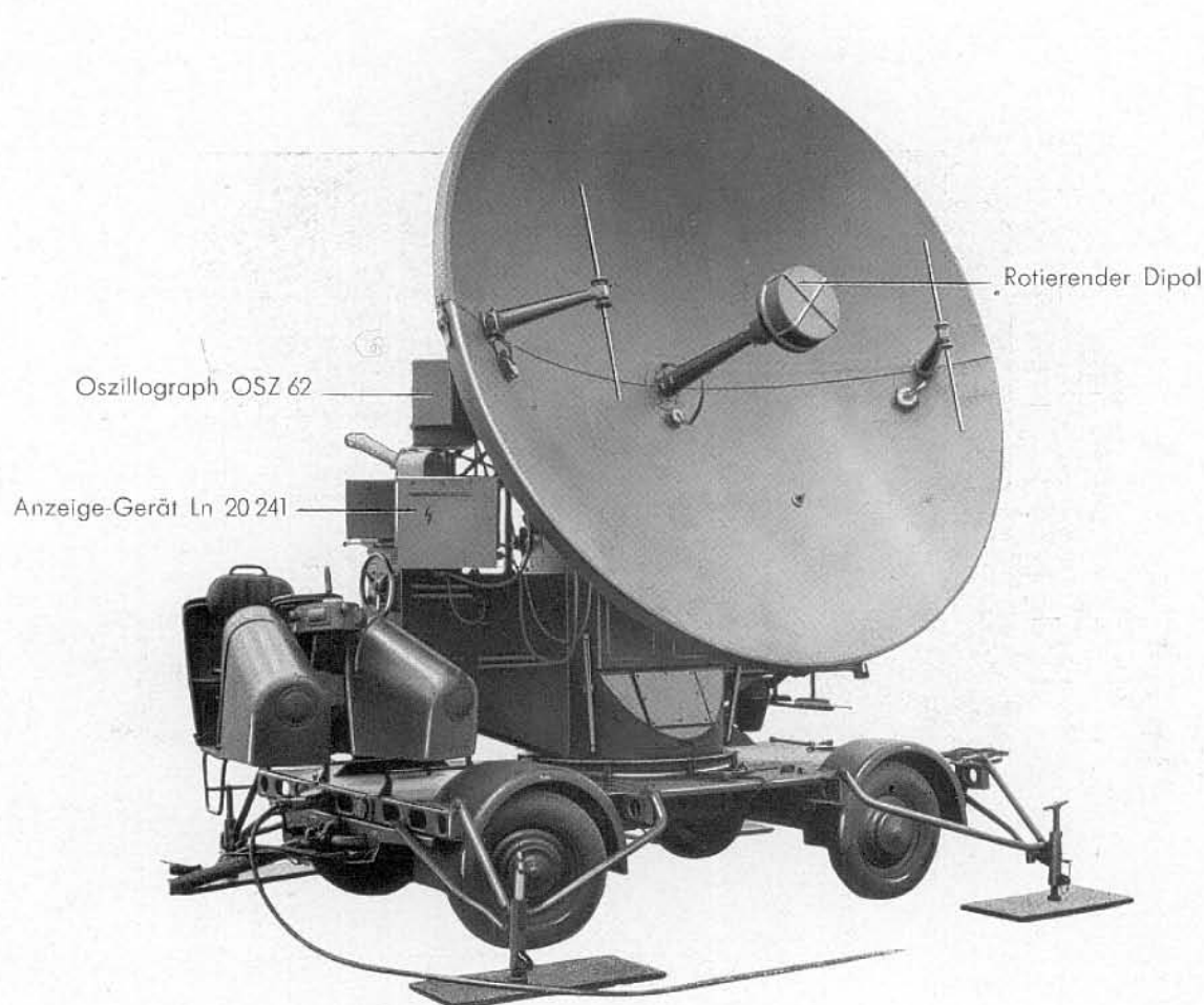
Abb. 6. Funk-Sende-Empfangsgerät FuSE 62 C
