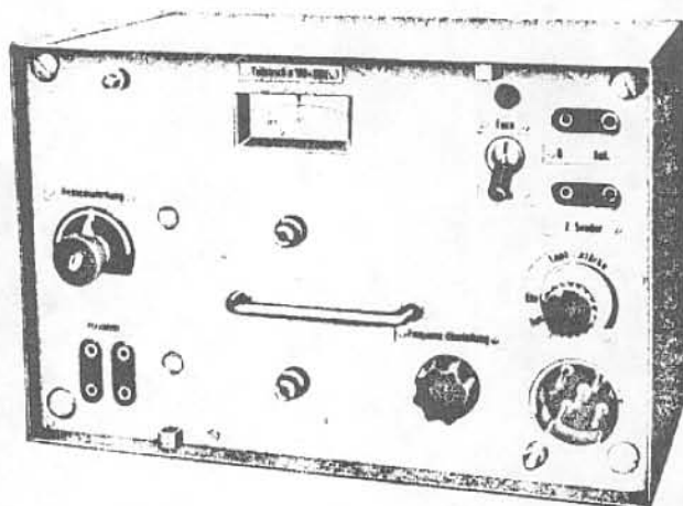
Vorderansicht des Empfängers E 433 Ba.
