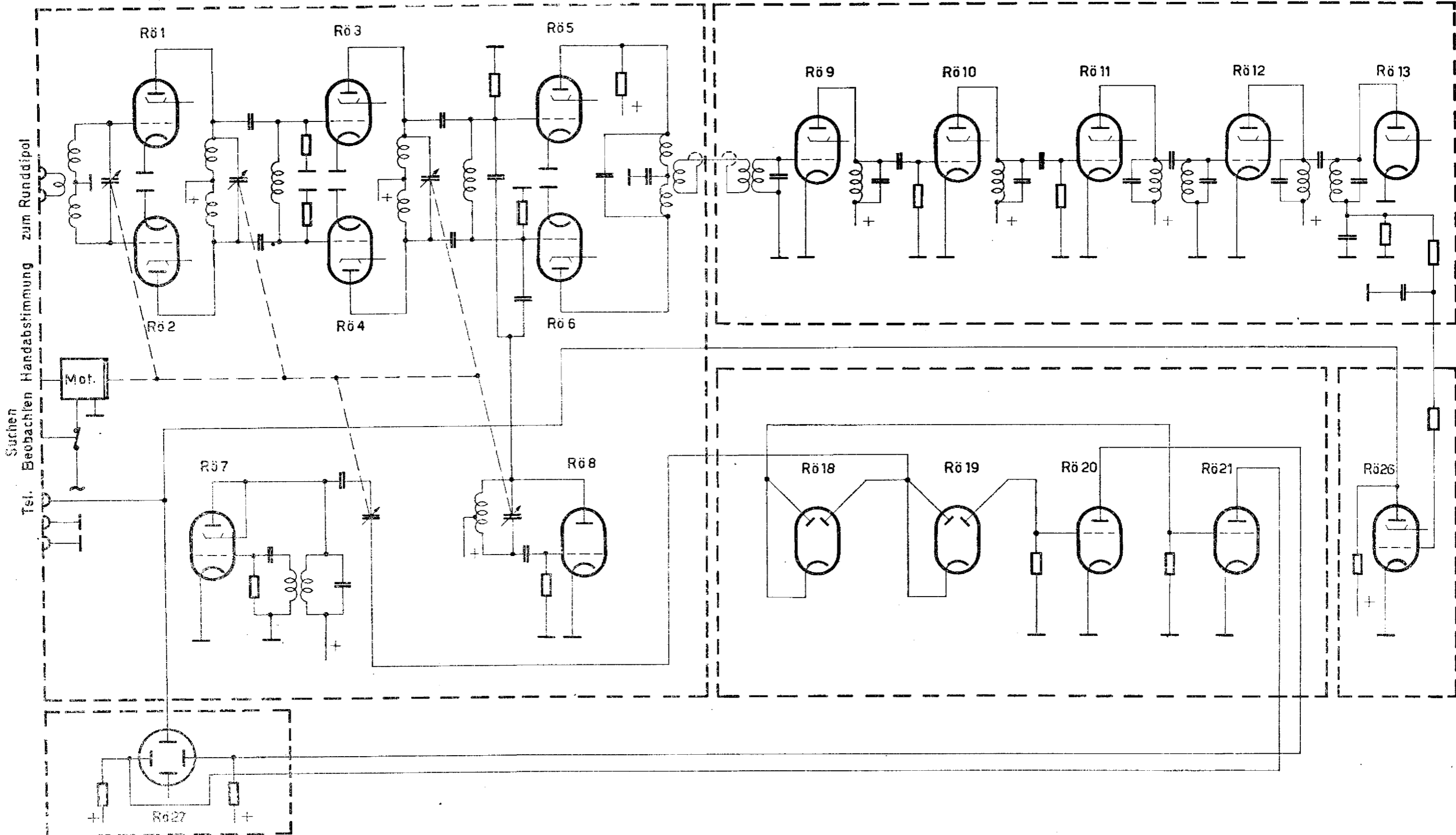
Prinzipschaltbild
