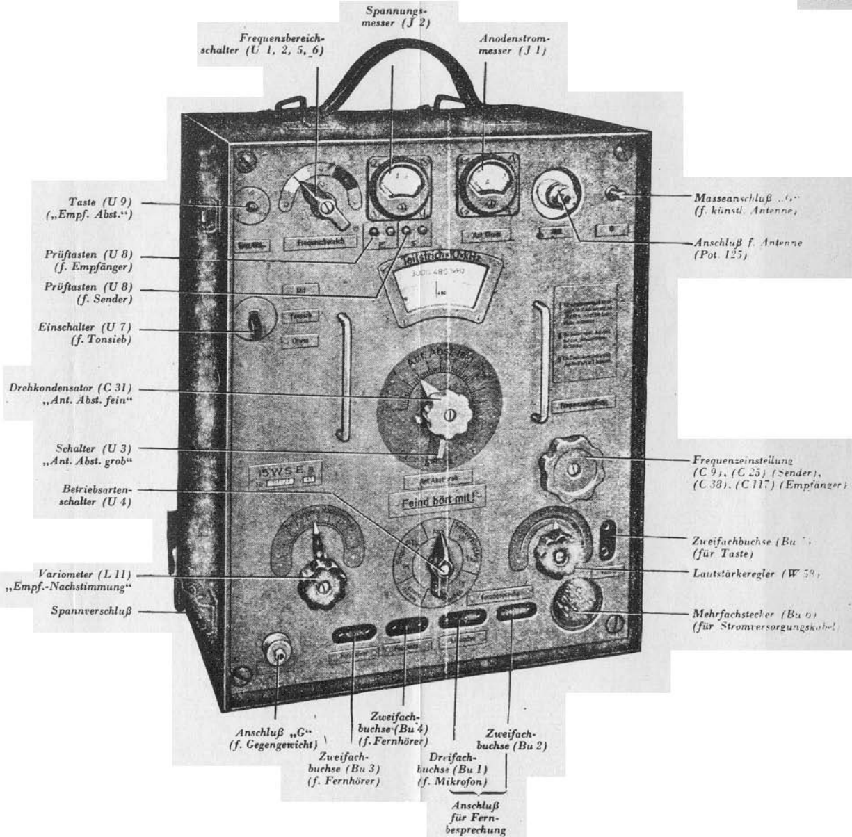
15 Watt Sender-Empfänger a (Deckel abgenommen)
