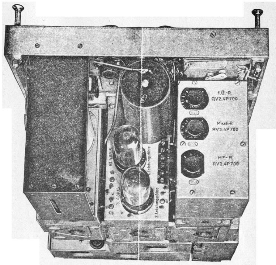
Sender-Empfänger, Ansicht von oben
