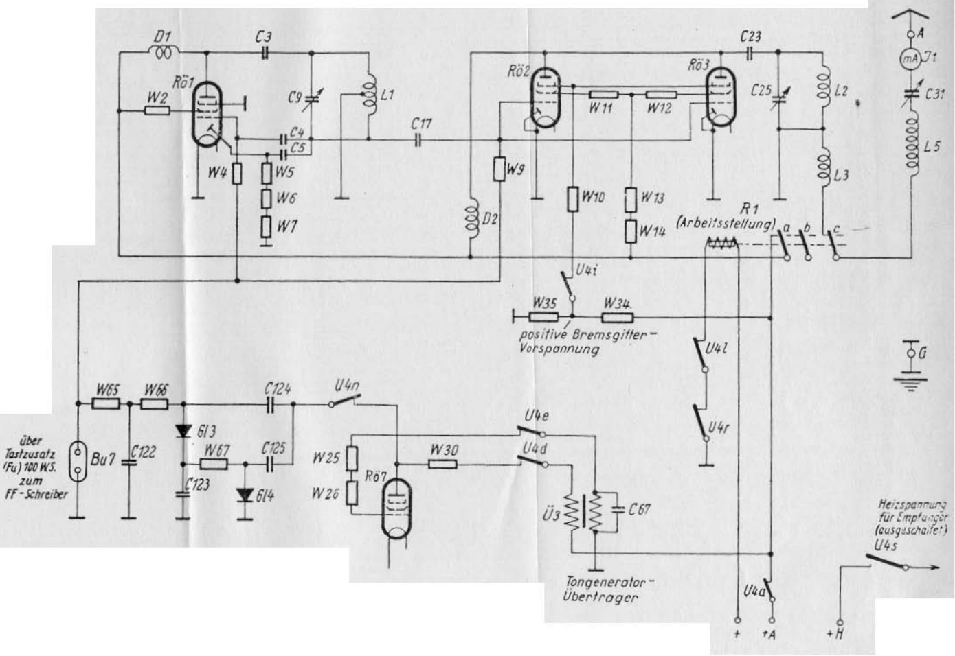
Grundsätzliches Schaltbild für Betriebsart „FF-Schreiber“ (Senden)
