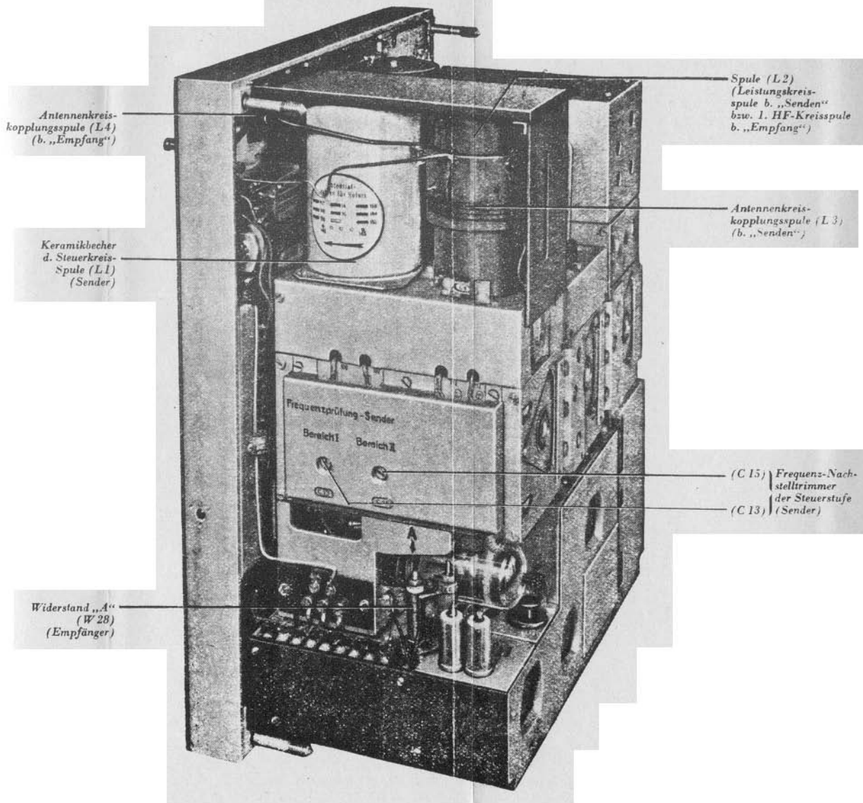
Rechte Seitenansicht des Sender-Empfängers
