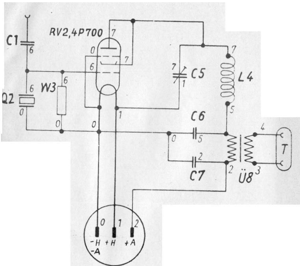
Schaltbild des Prüfers SE 15 b
